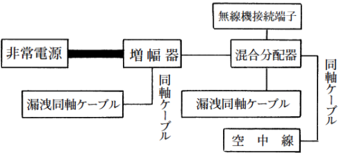
第26ー3図 耐火・耐熱保護配線の範囲
